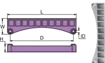
OMC P
