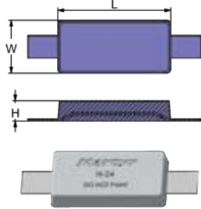
BOLT-ON
