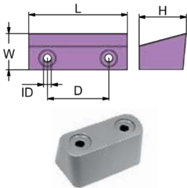
OMC COBRA
