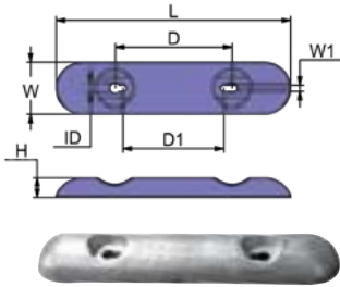
BOLT-ON
