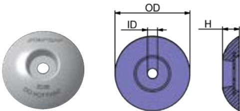
BOLT-ON
