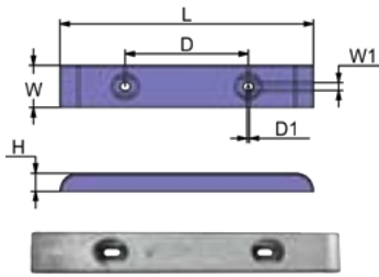
BOLT-ON
