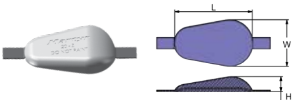
BOLT-ON
