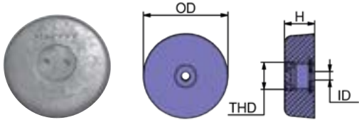
BOLT-ON
