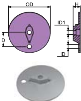
BRAVO4 225-250 HP
