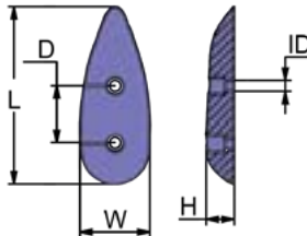
BOLT-ON
