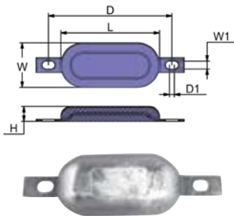
BOLT-ON
